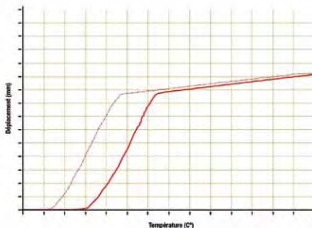
Déplacement du couvercle en fonction de la température du THERMOSTAT FAE
